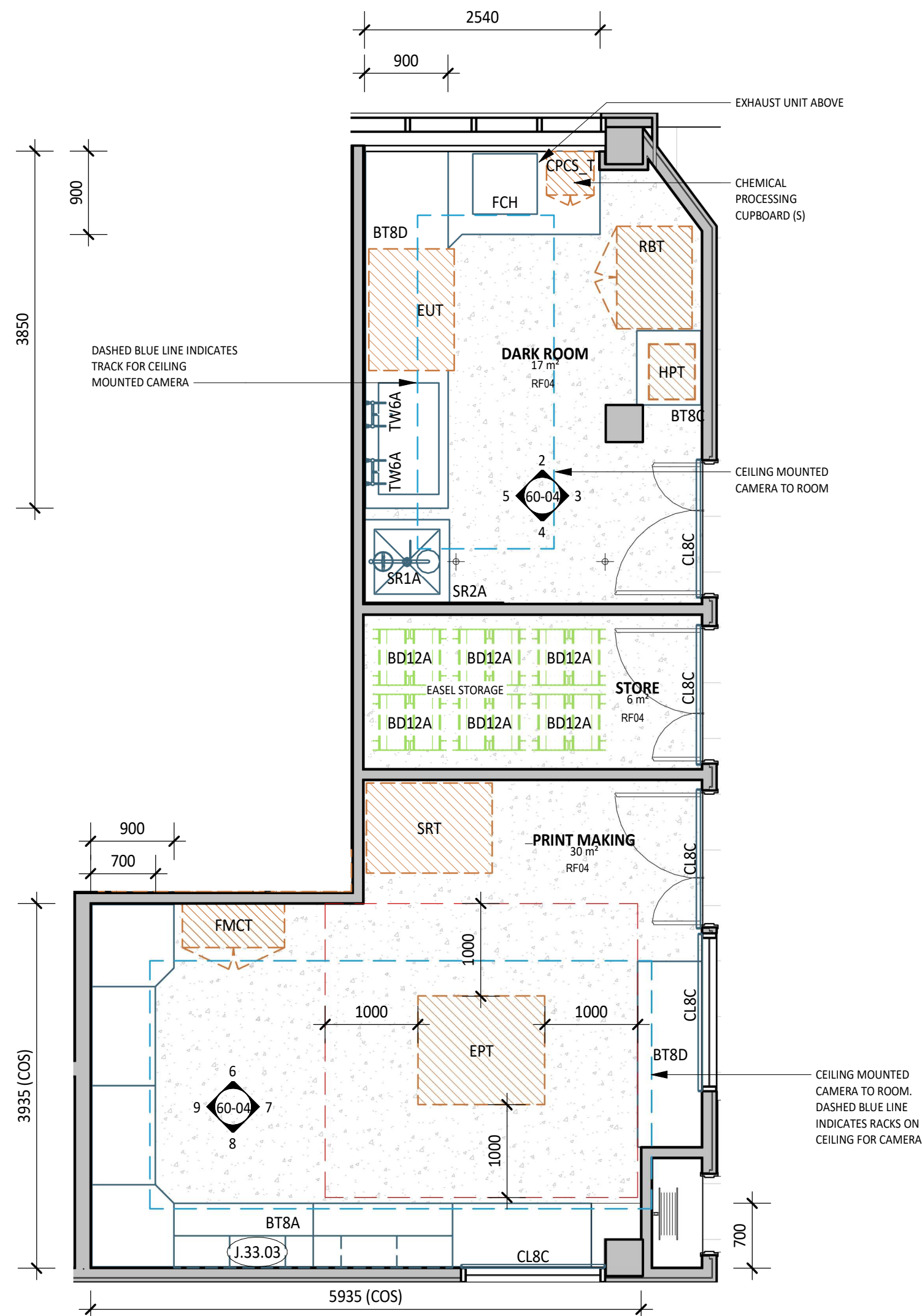
1 PLAN DETAIL 1 : 50
